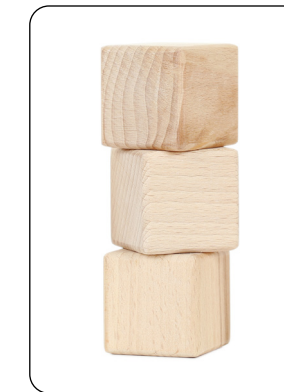
opaque object
